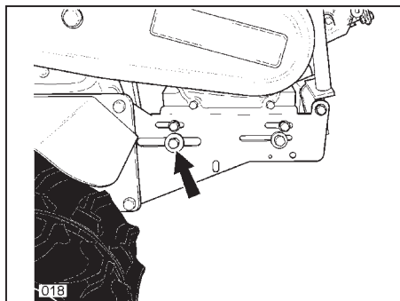
Pennen koppelingshendel
