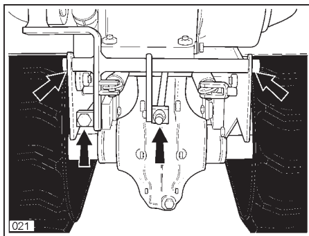
Pernos palanca frenos
