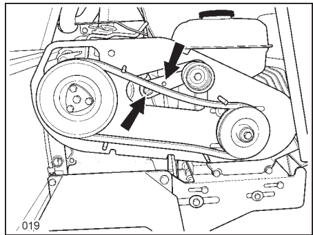
Riemenspanner
