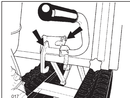
Alavanca e mecanismo de bloqueio da caçamba
