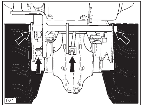
Bolzen Bremshebel
